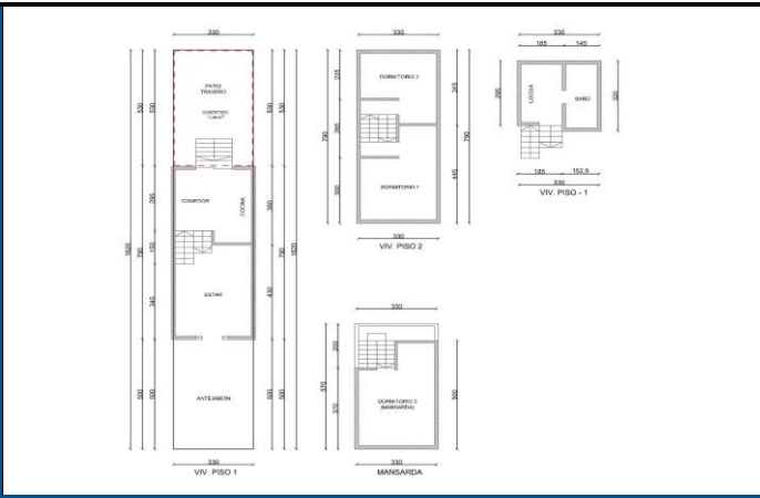
Planificación
